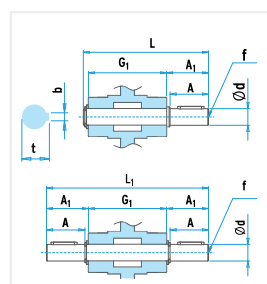
CRV/CMRV | Albero lento applicato / Output shaft
