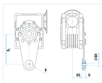
CRV-E/CMRV-E | Braccio di reazione / Torque arm
